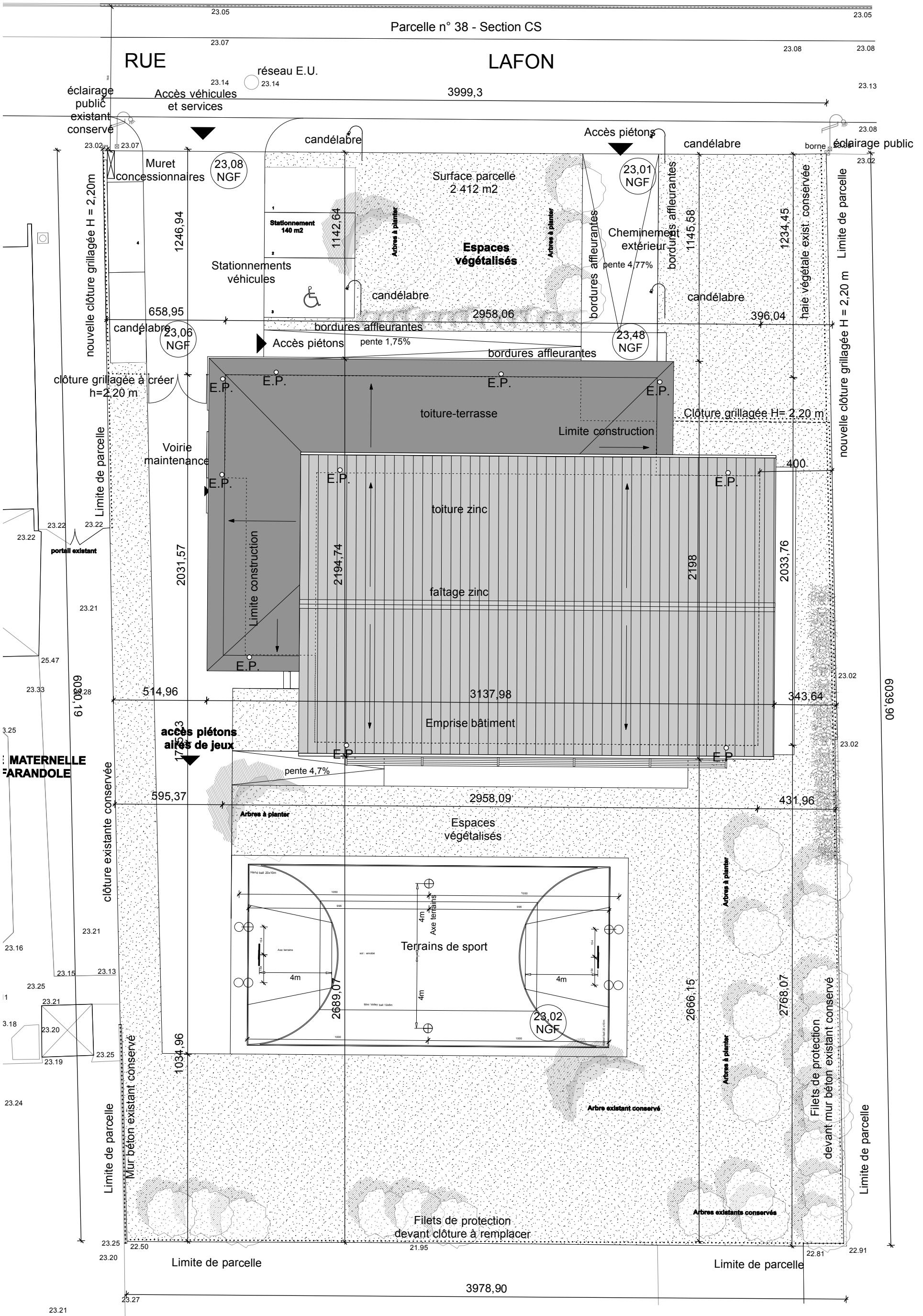
Plan de masse - échelle 1 / 200
